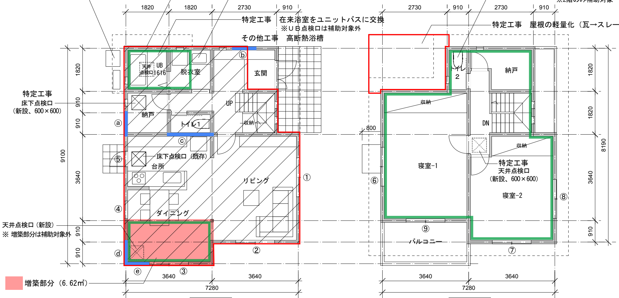
1階平面図
