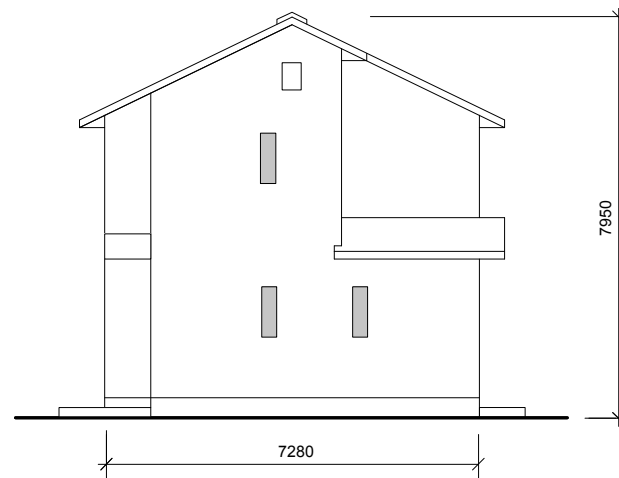
北立面図
